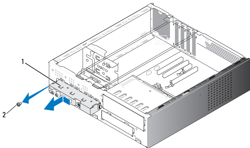
1 输入 / 输入面板 2 螺钉
