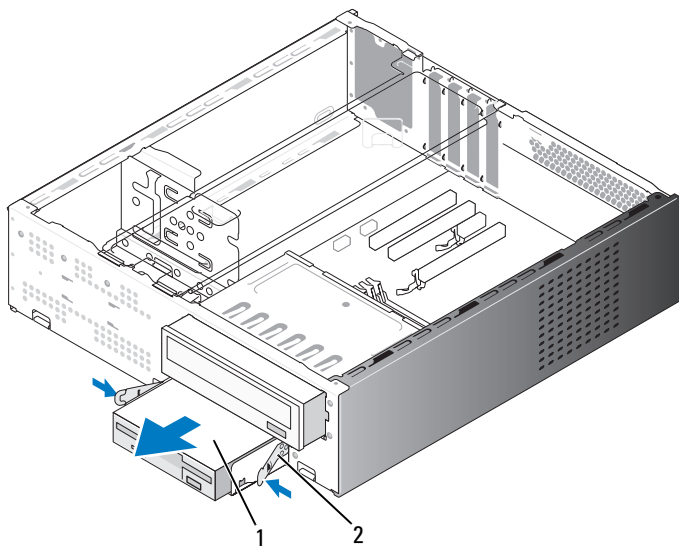
1 软盘驱动器 2 弹簧夹 (2)
