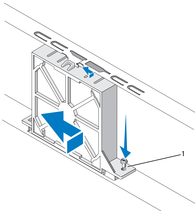
1 螺钉
