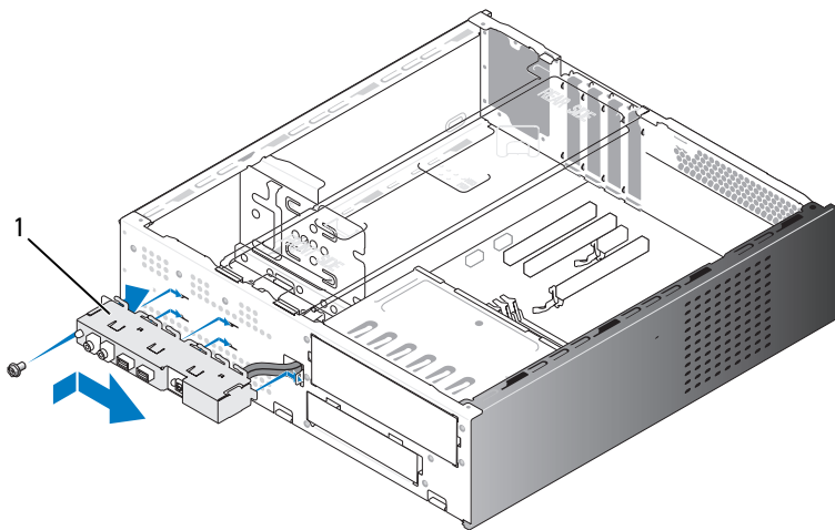
1 输入 / 输入面板
