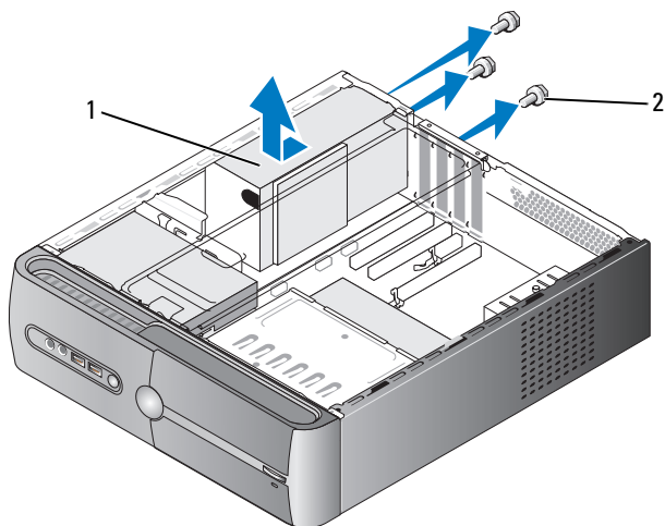
1 电源设备
