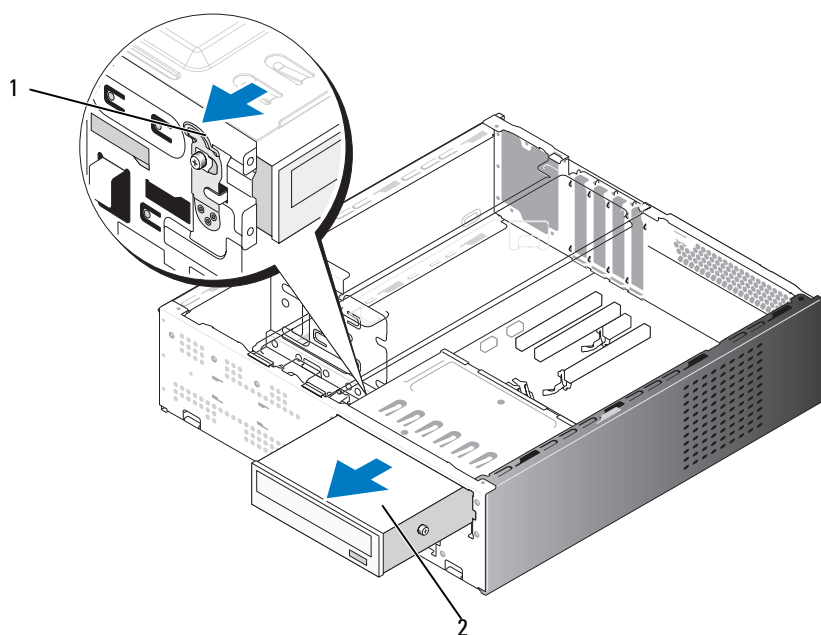
1 光盘驱动器托架释放拉杆 2 光盘驱动器
