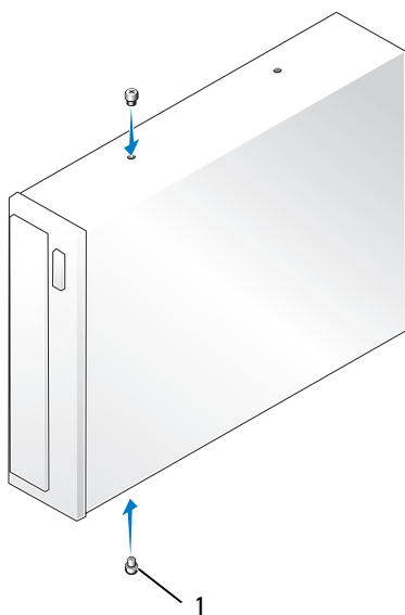
1 轴位螺钉 (2)
